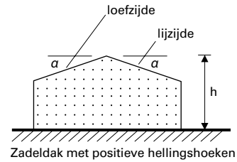
Zadeldak met positieve hellingshoeken
