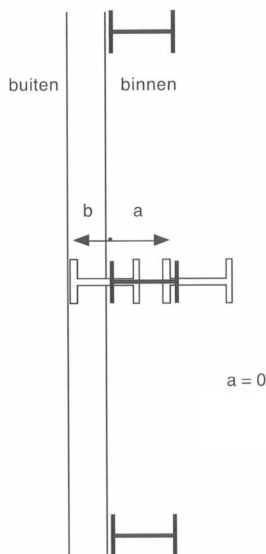
Aanvullende tolerantie achterconstructie bij sandwichpanelen ( a = 0 ; b = conform NEN-EN 1090-2, Klasse 2)
